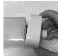
4: Séparez le capuchon du corps du tube en veillant à ne pas égarer ou abîmer l'anneau de silicone waterproof.
